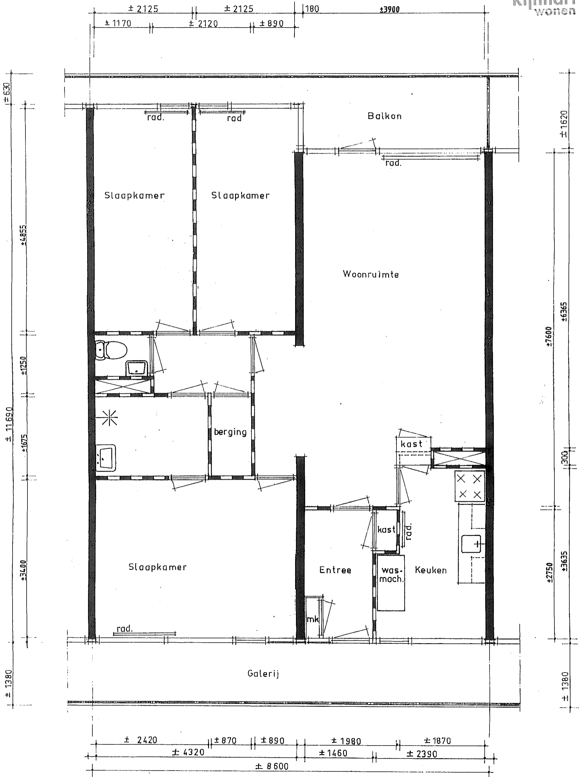
Plattegrond 1:50
